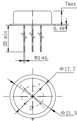
图 2 HC-40U
