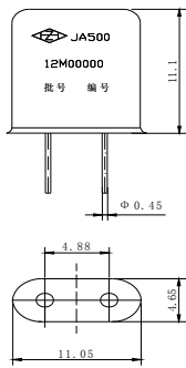
图 1 HC-49T
