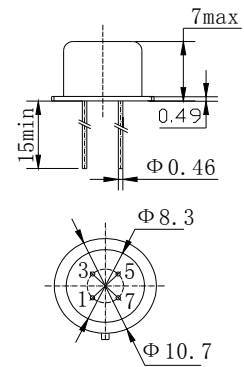
图 3 HC-35U (T0-5)
