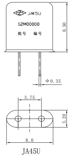
外形尺寸图
